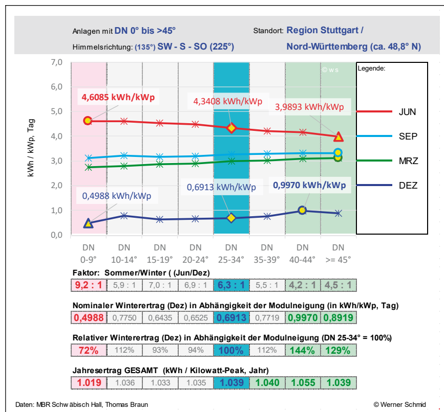
Bild 2: Durchschnittlicher PV-Tagesertrag in kWh/Kilowatt-Peak
