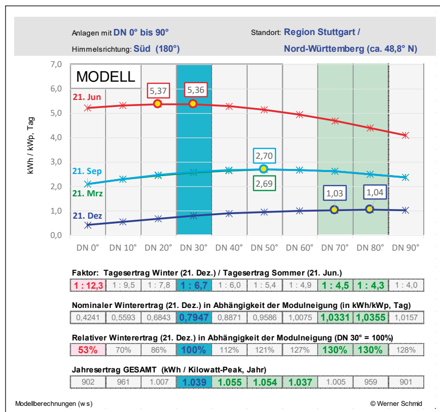
Bild 3: Simulierter durchschnittlicher PV-Tagesertrag in kWh/Kilowatt-Peak
