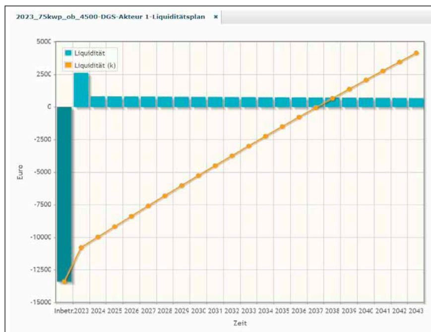
Bild 2: Wirtschaftlichkeit Volleinspeisung
