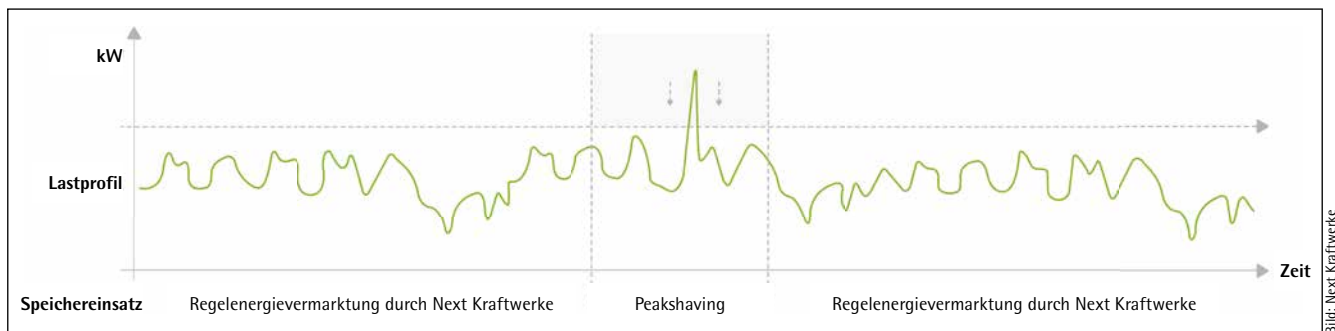
Bild 5: Schematische Darstellung eines Speichereinsatzes mit Peakshaving und Regelenenergievermarktung.
