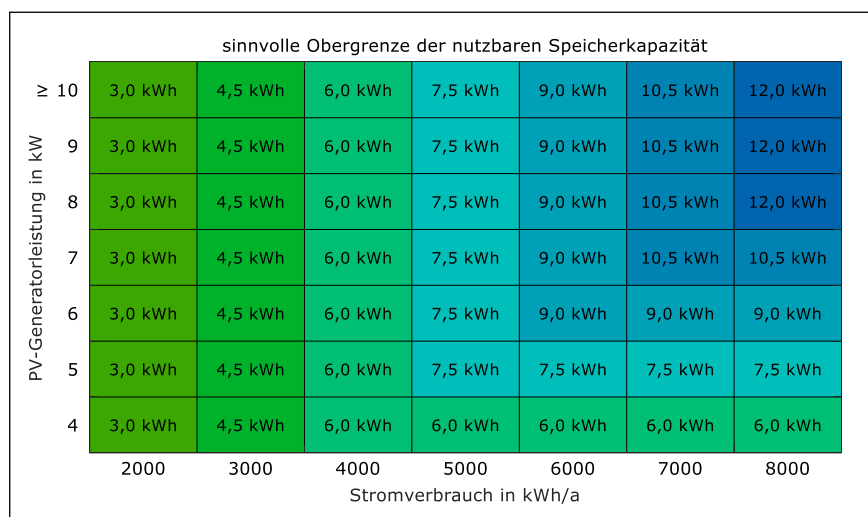
Bild 1: Empfohlene Obergrenze der nutzbaren Speicherkapazität in Einfamilienhäusern, die von der Größe der PV-Anlage und von der Höhe des jährlichen Stromverbrauchs abhängt.
