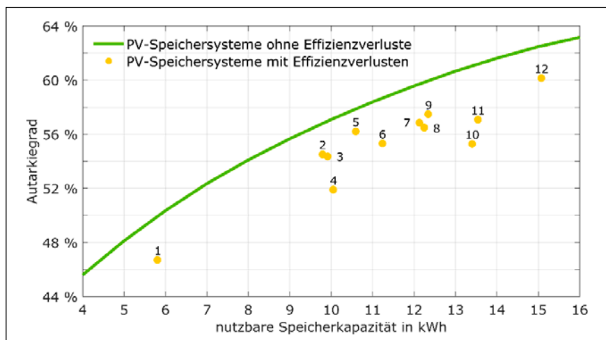
Bild 2: Einfluss der Effizienzverluste unterschiedlich dimensionierter PV-Speichersysteme auf den Autarkiegrad eines Einfamilienhauses mit Wärmepumpe und Elektroauto (PV-Nennleistung: 10 kW, Stromverbrauch: 9.364 kWh/a).
